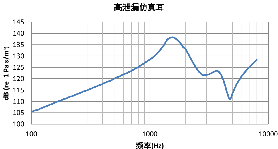
图一 声学阻抗典型曲线
